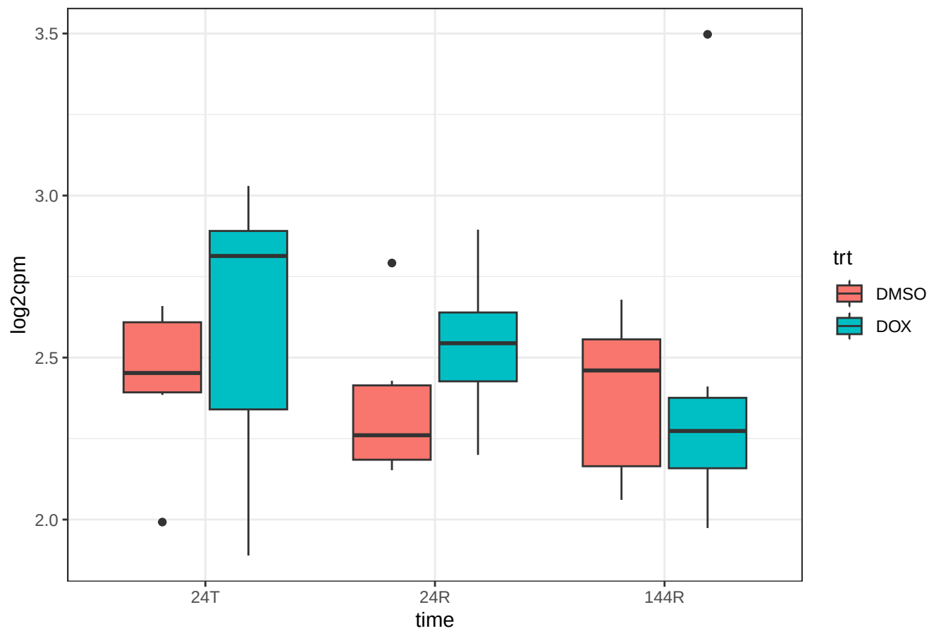
gene 8187 ZNF239
